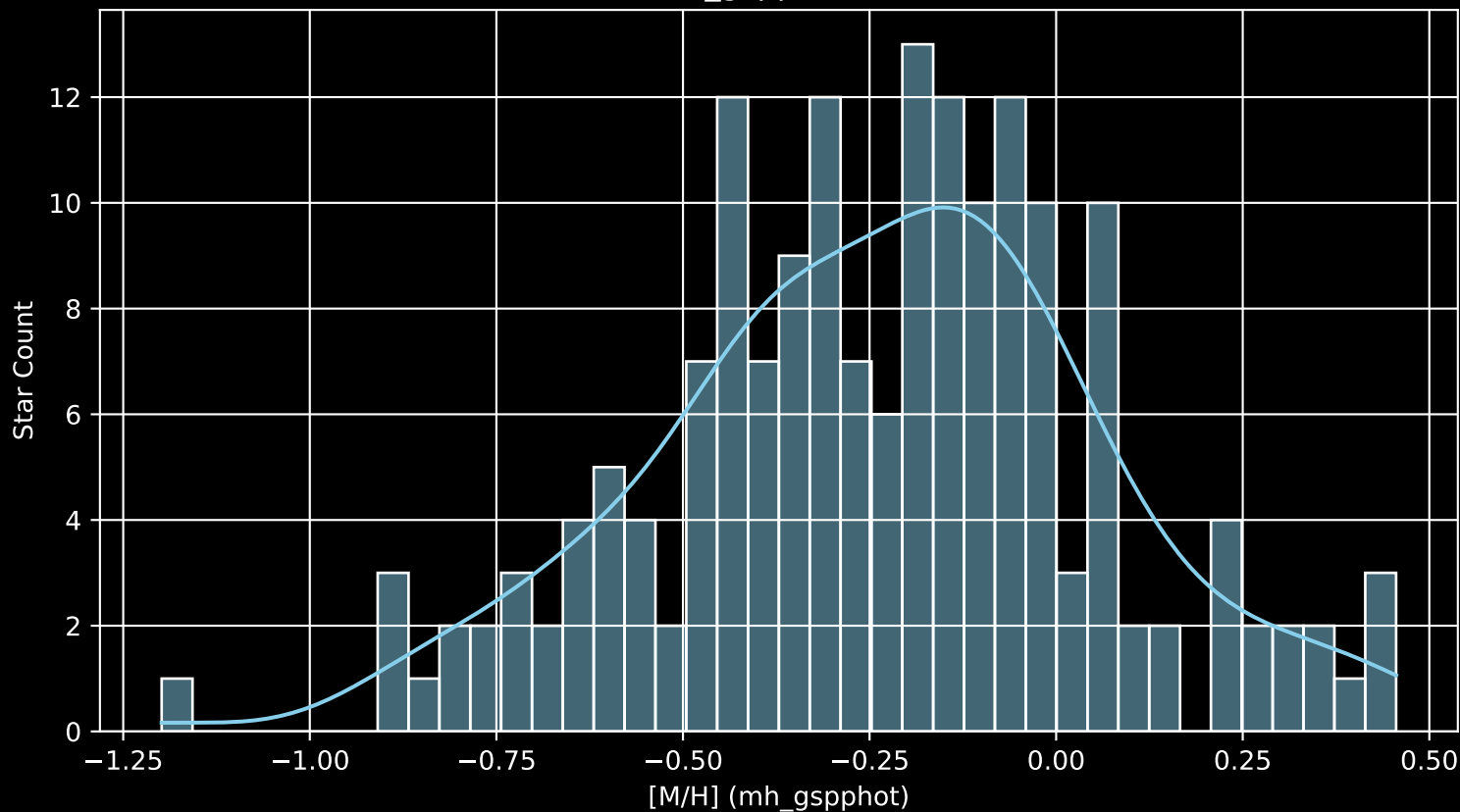
APOGEE DR17 Field: [233+36 MGA [M/H] (mh_gspphot) (n= 177)
